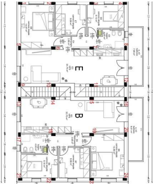
piano piano primo - SX
