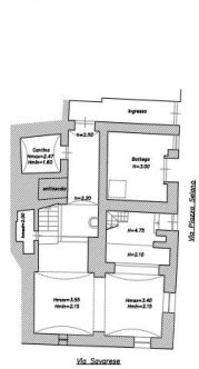
Pianta Piano terra scala 1:100
