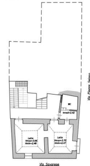
Pianta Piano Secondo scala 1:100
