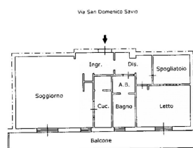
PIANO SECONDO h = 2,70 mt
