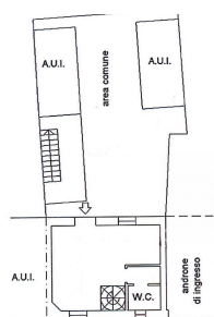
VIA NAZARIO SAURO PIANTA PIANO TERRA H=270
