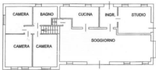
PIANTA PIANO RIALZATO H = 2,80
