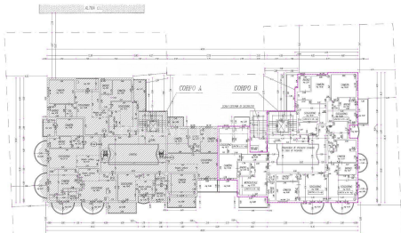
PIANTA PIANO 3°
