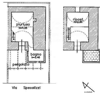
PIANTA PIANO TERRA PIANTE PIANO AMMEZ.
