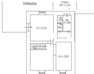
PIANO PRIMO
